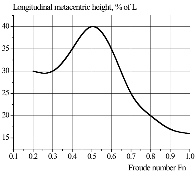
Slika 8 Primjer uzdužne metacentarske visine predloženog SWATH-a
