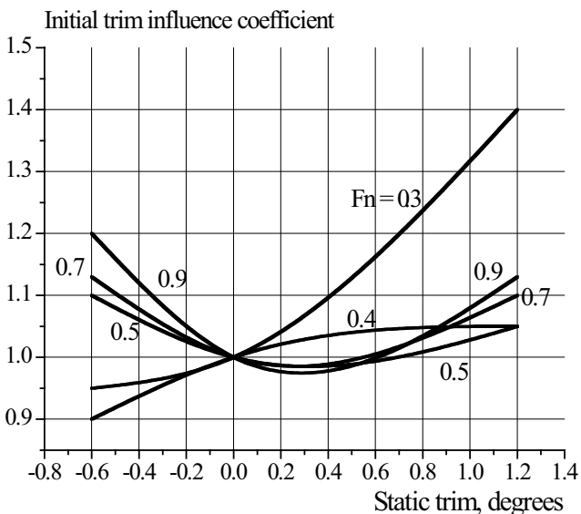
Slika 2 Primjer utjecaja početnog trima na koeficijent preostalog otpora C_r tradicionalnog SWATH-a
