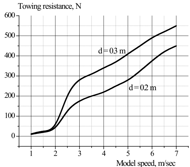
Figure 6 Towing resistance of the model tested at two draughts Slika 6 Otpor tegljenja modela izmjeren za dva gaza
