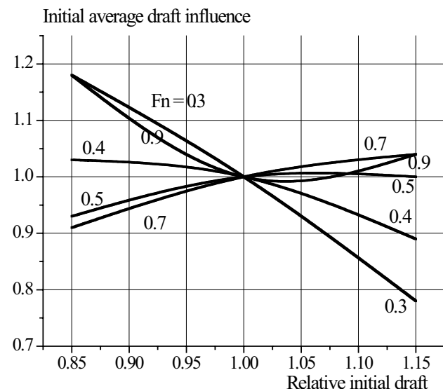
Slika 4 Primjer utjecaja početnog srednjeg gaza na koeficijente preostalog otpora tradicionalnog SWATH-a (konstantna istisnina)
