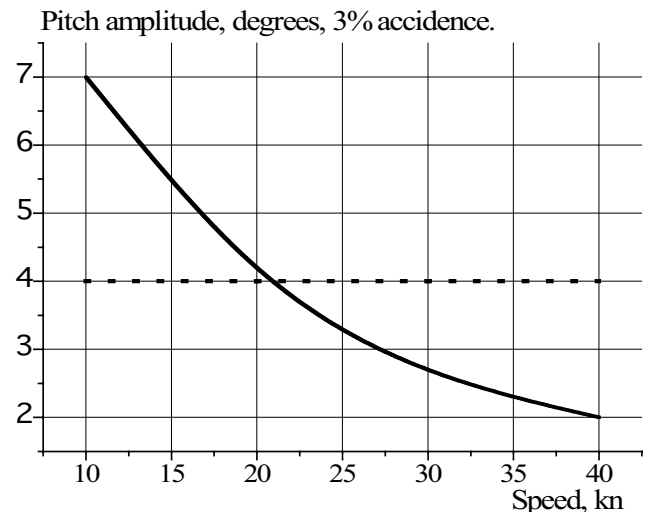
Slika 14 Amplituda posrtanja na valovima u pramac ophodne SWATH korvete
