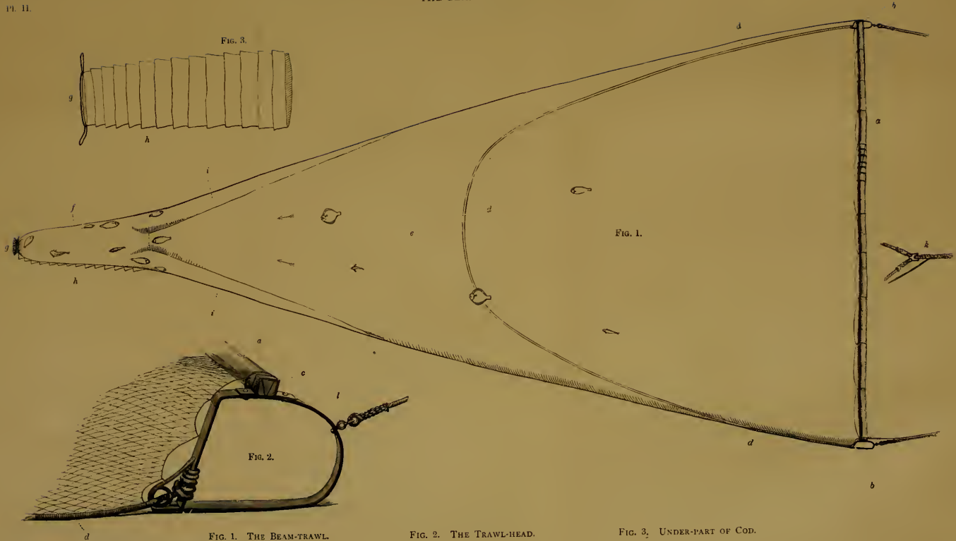
FIG. 1. THE BEAM-TRAWL.
